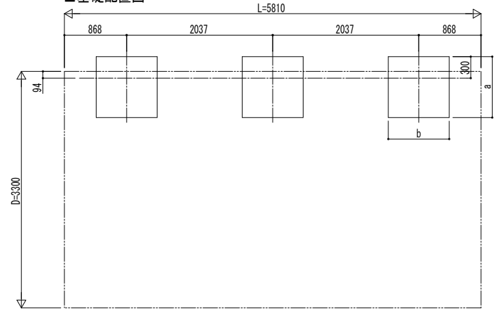
■基礎配置図
