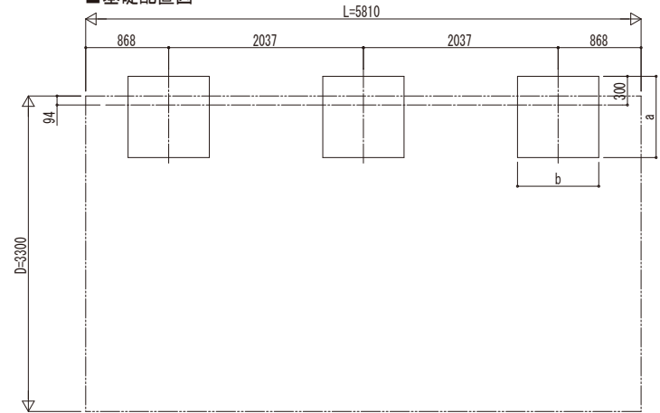
■基礎配置図
