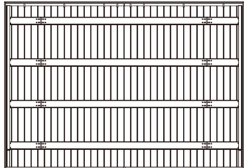
■姿図
