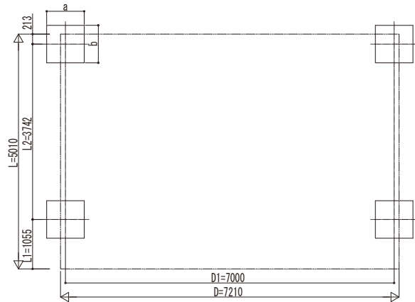
■基礎配置図
