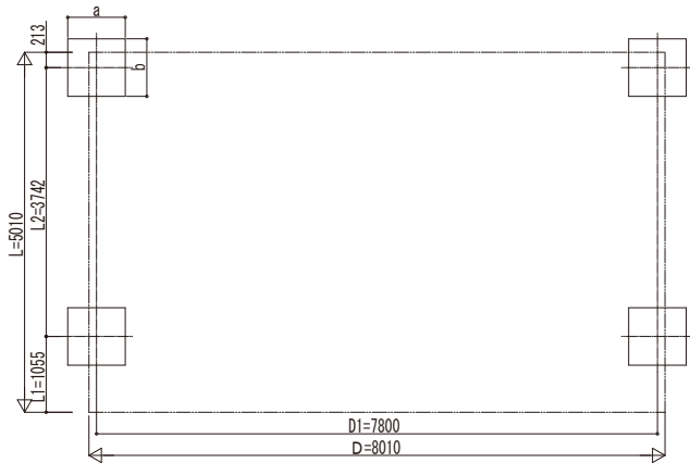
■基礎配置図
