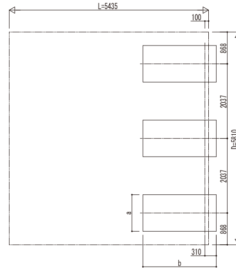
■ 基礎配置図
