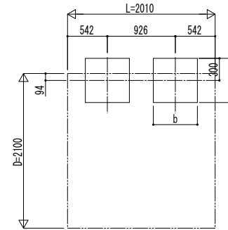
■ 基礎配置図
