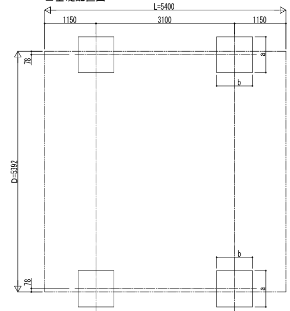
■ 基礎配置図
