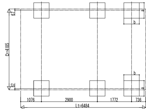
■基礎配置図
