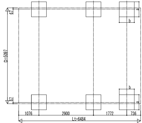
■ 基礎配置図
