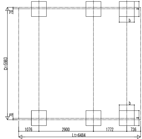
■ 基礎配置図
