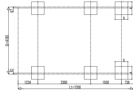
■ 基礎配置図
