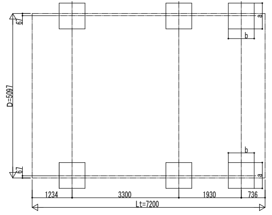
■ 基礎配置図
