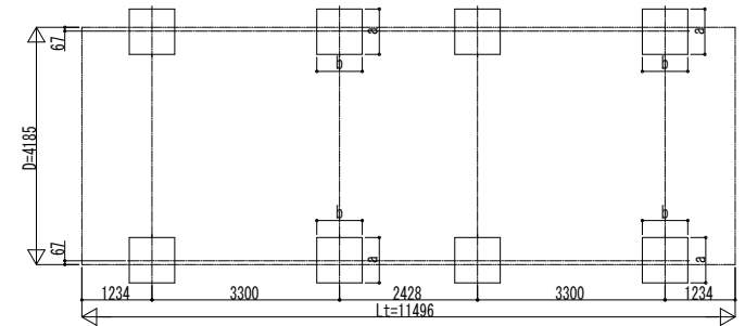
■ 基礎配置図
