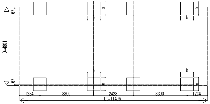
■ 基礎配置図
