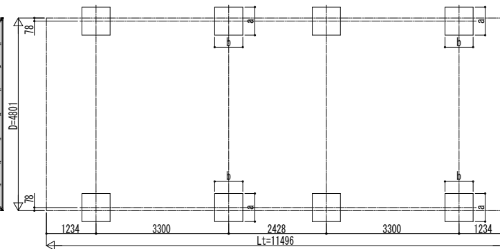
■ 基礎配置図
