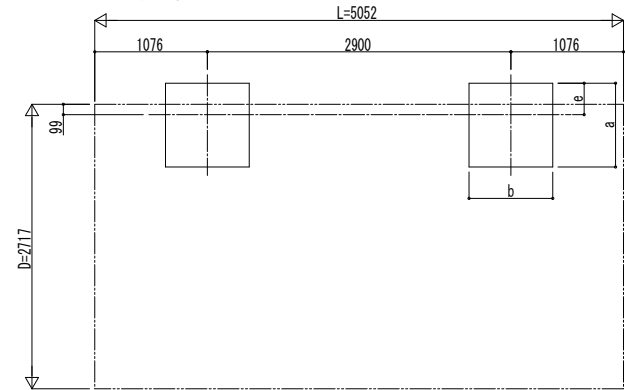
■基礎配置図
