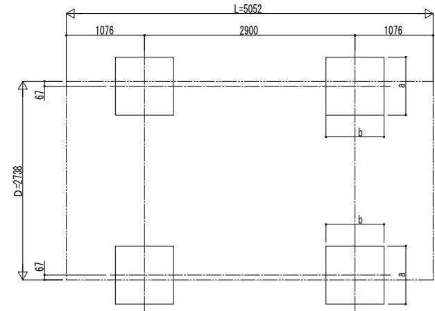
■ 基礎配置図
