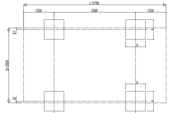
■ 基礎配置図
