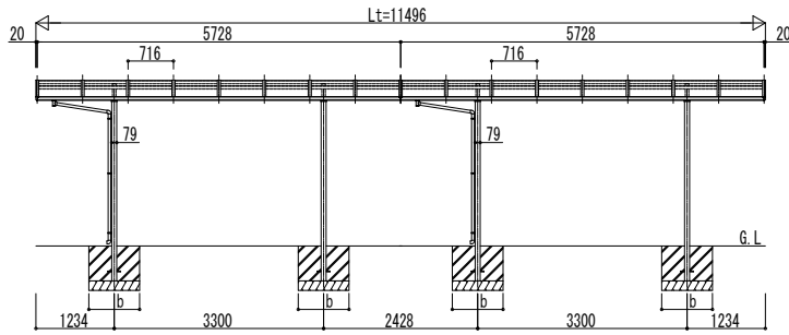
■ 基礎寸法表
