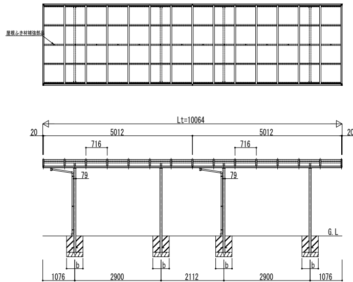
■ 姿図
