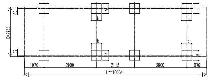
■ 基礎配置図
