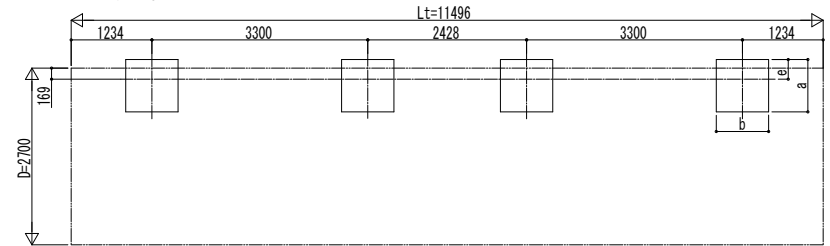
■ 基礎配置図
