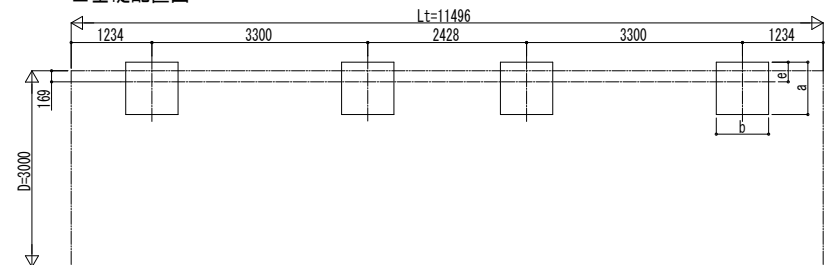
■ 基礎配置図
