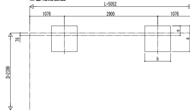
■ 基礎配置図
