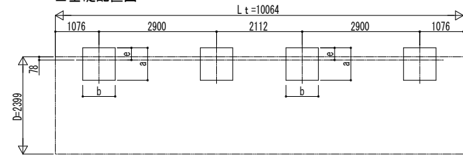
■ 基礎配置図
