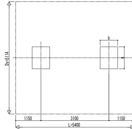
■ 基礎配置図
