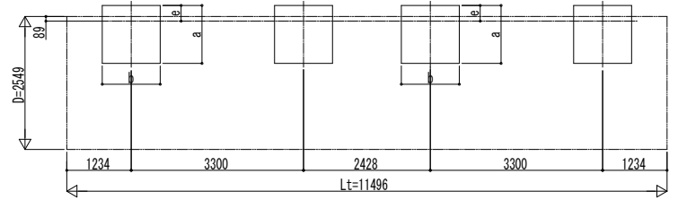
■ 基礎配置図
