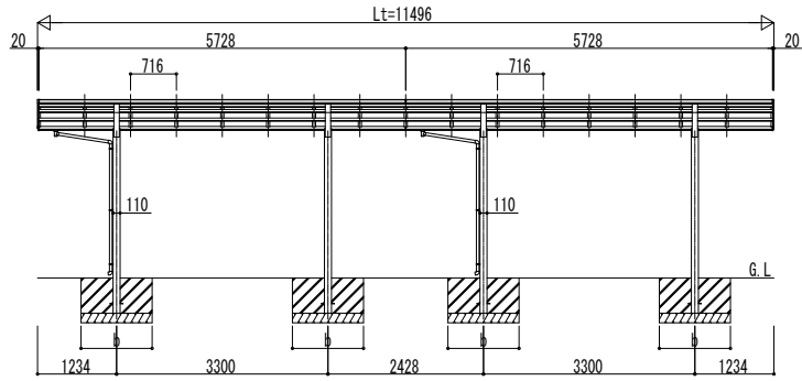
■ 基礎寸法表
