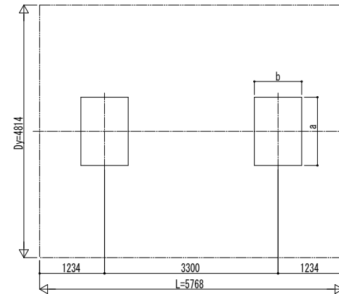
■ 基礎配置図
