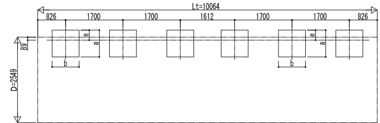
■ 基礎配置図
