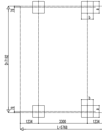
■ 基礎配置図
