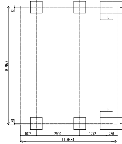
■ 基礎配置図
