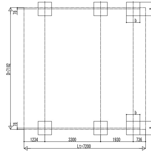
■ 基礎配置図
