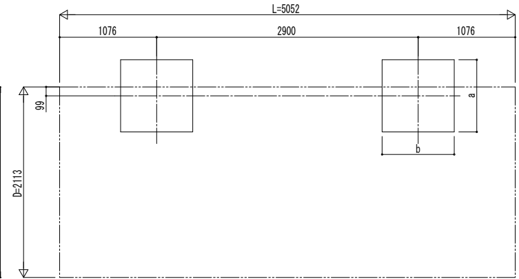
■ 基礎配置図
