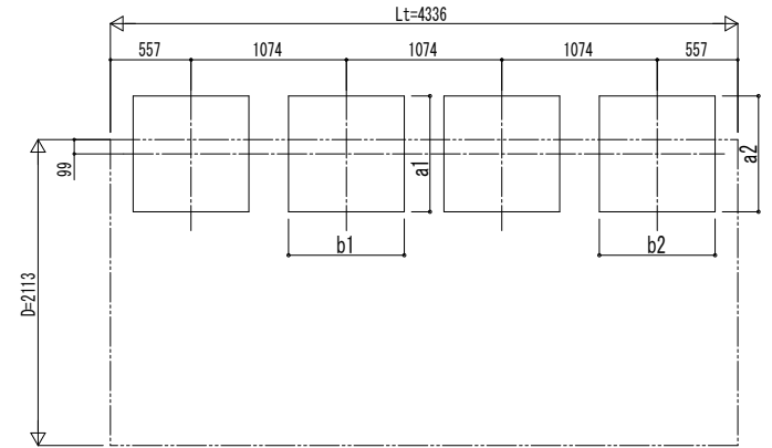
■基礎配置図
