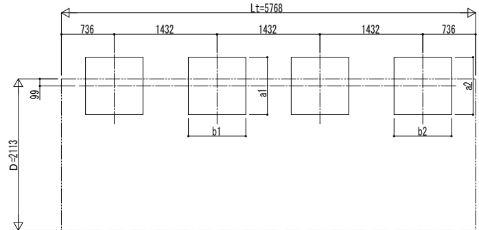
■ 基礎配置図
