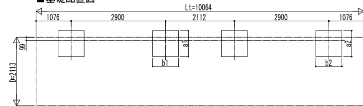
■ 基礎配置図
