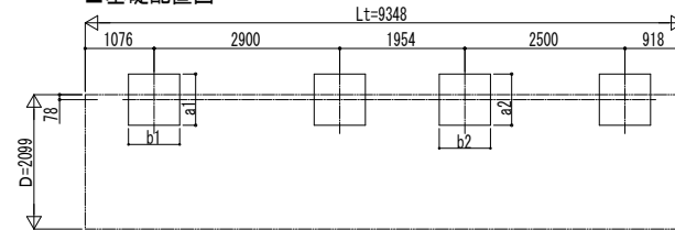
■ 基礎配置図
