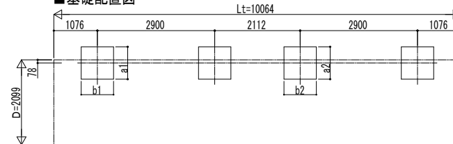
■ 基礎配置図
