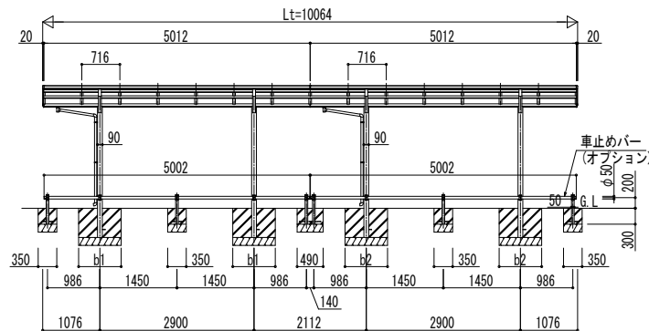
■ 基礎寸法表
