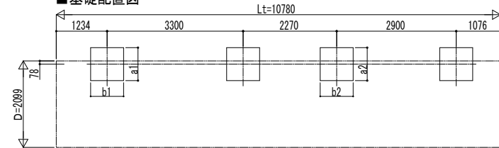
■ 基礎配置図
