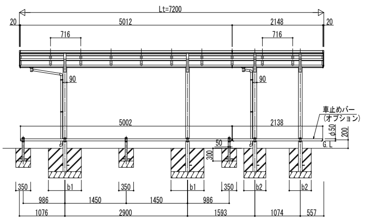
■ 基礎寸法表
