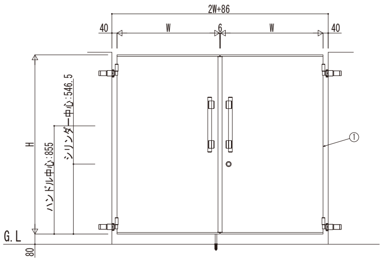
打掛錠1型の場合
