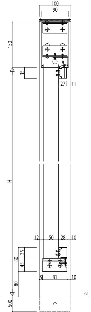
断面図
