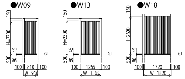
姿図
