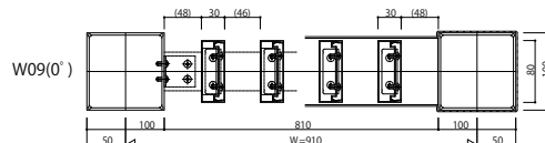
移動柱納まり
