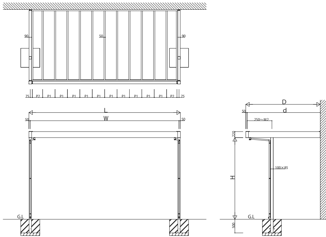
本図は【関東間 5427 H30】を表す。
