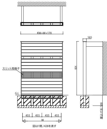
スリット + スリット格子
