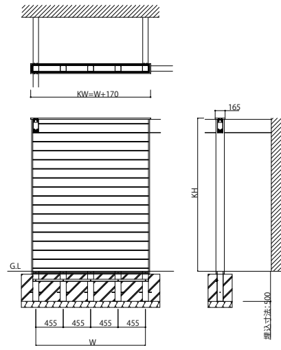
梁正面接合 + 梁側面接合
