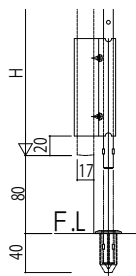
落し錠部縦断面図
