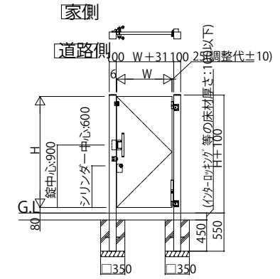
片開き 外観姿図 (1:20)
