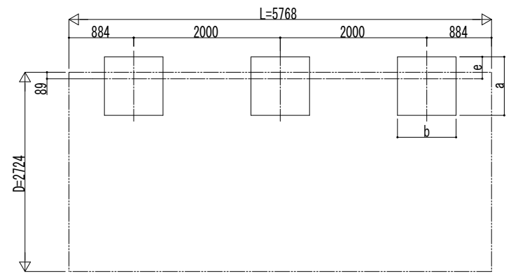
■ 基礎配置図
