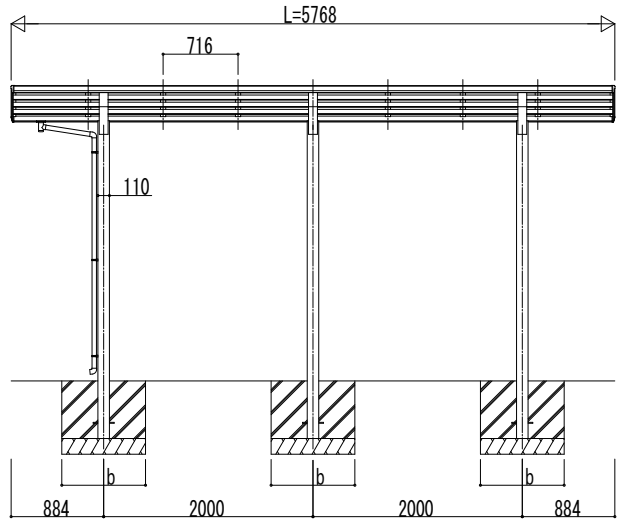
■ 基礎寸法表
