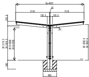
●22-21・21 車止めバー付き (オプション)
