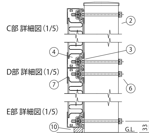
パネル (遮音タイプ H1m) 詳細図 (1/25)
