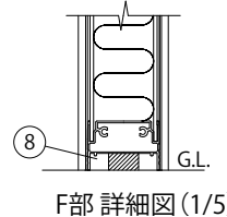
F部詳細図(1/5)
