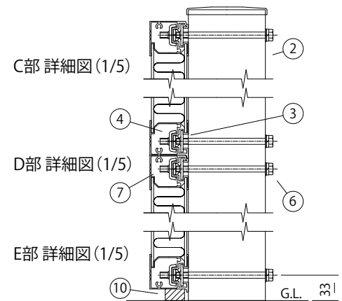
パネル (吸音タイプ H1m) 詳細図 (1/25)
